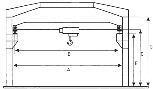
Typ B
