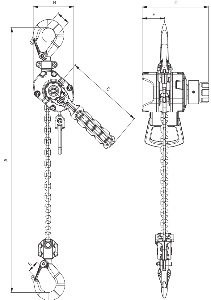
PAH 500 – 3.000 kg
