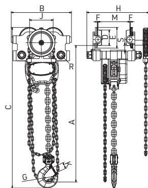
LHT-G 3.000 kg
