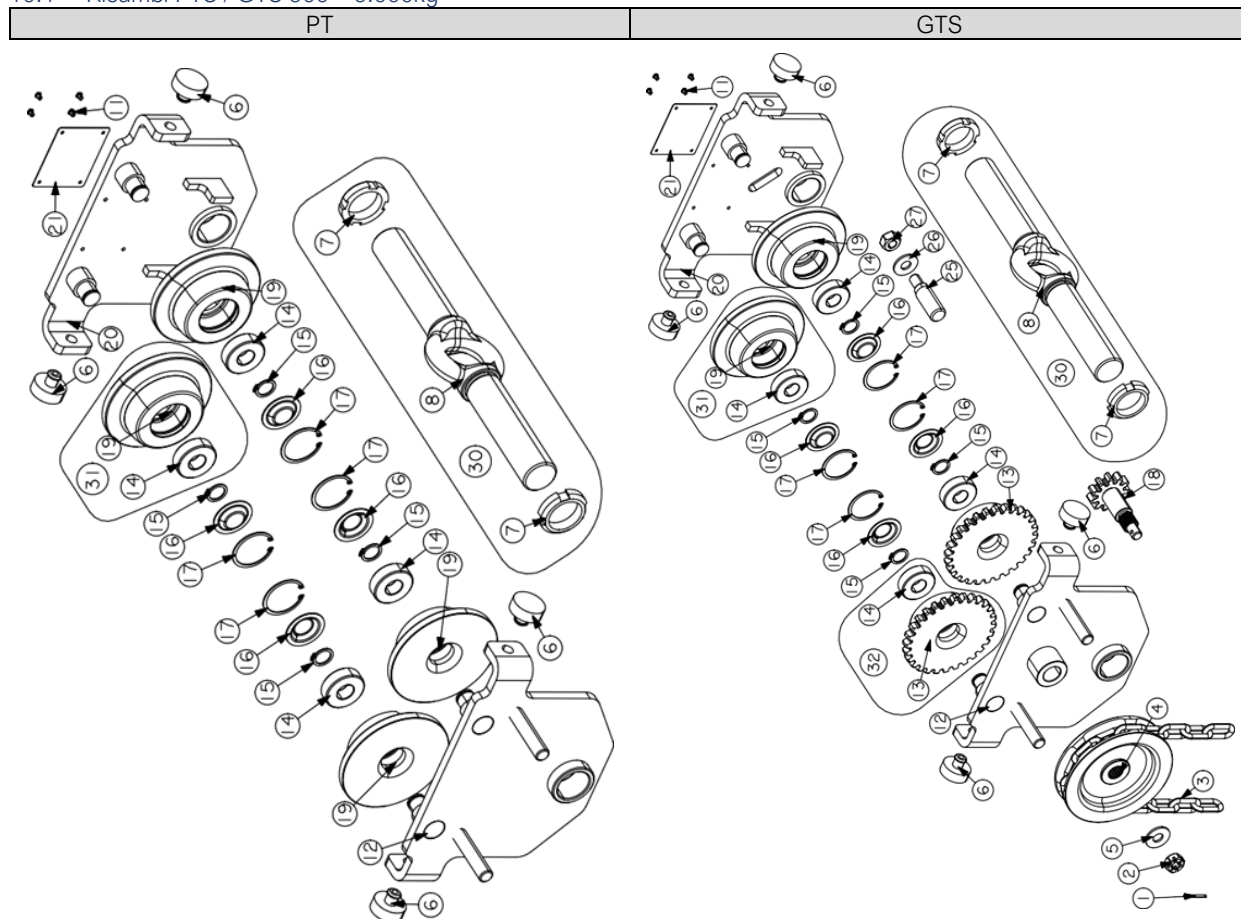
Tavolo 6 Ricambi PTS / GTS 500kg – 5.000kg
