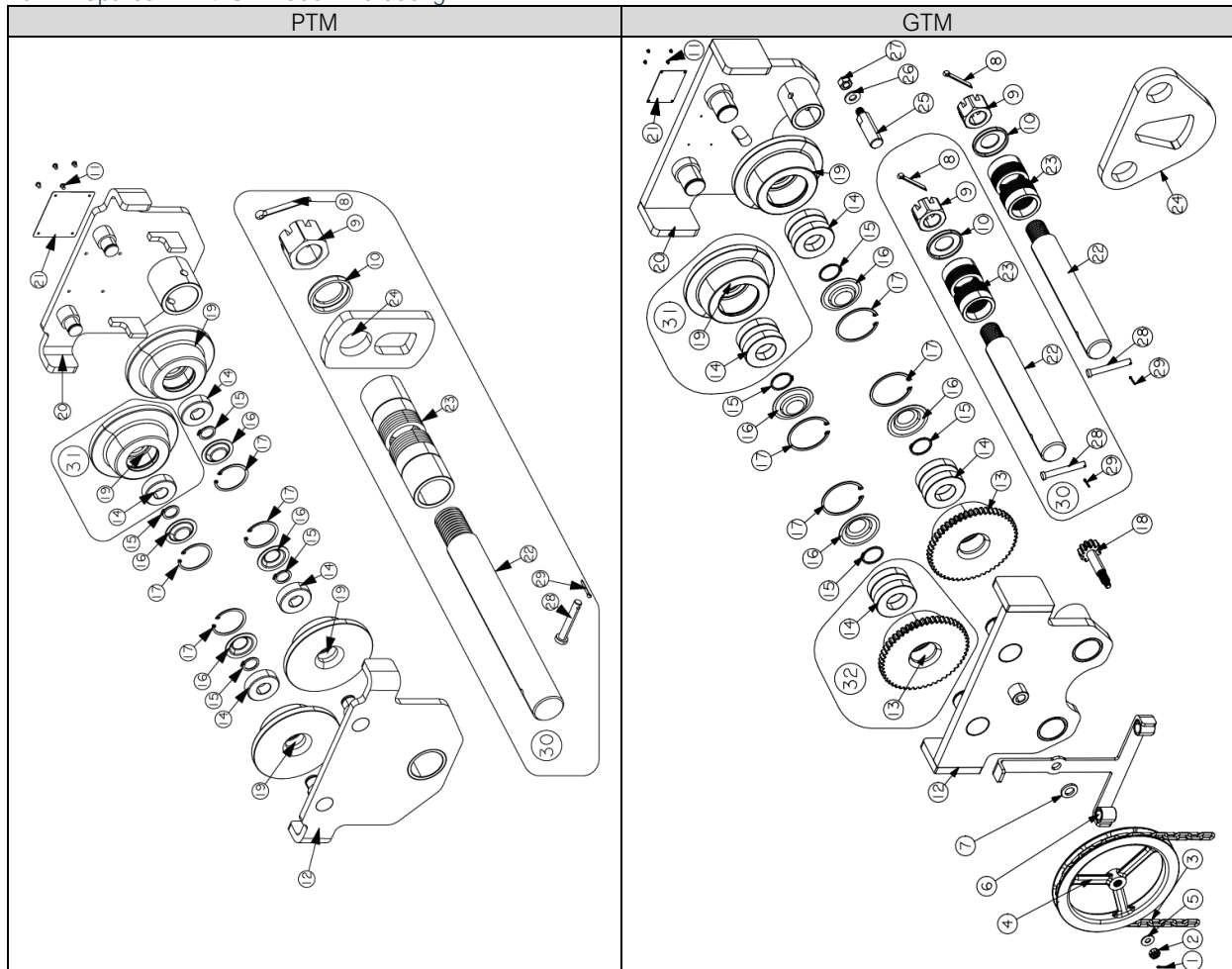
Tafel 6 Spares PTM / GTM 500kg – 20.000kg
