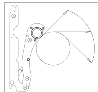
Abbildung 6 Seilandruckrolle PFW
