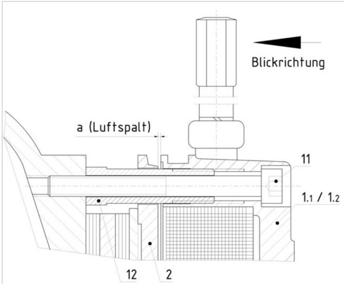
Abbildung 45 Bremsspieleinstellung Typ FDB / FDD
