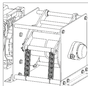
Abbildung 9 Seilandruckrolle PORTY
