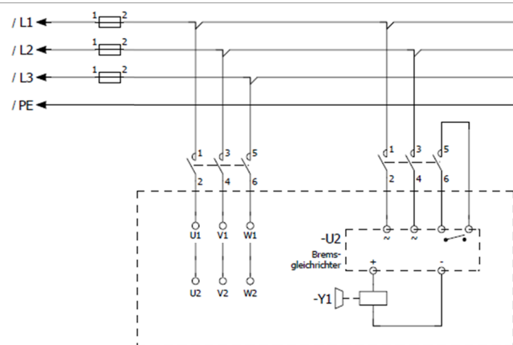
Abbildung 28 Anschluss-Beispiel
