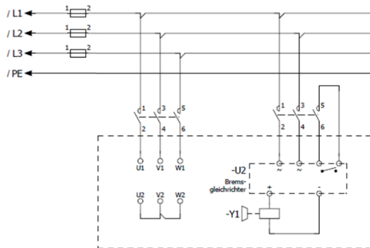
Abbildung 27 Anschluss-Beispiel
