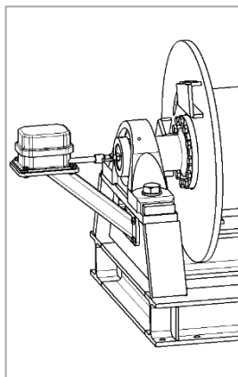
Abbildung 11 Spindelendschalter PHW
