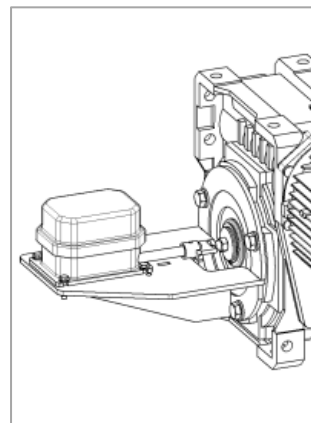
Abbildung 12 Spindelendschalter PORTY
