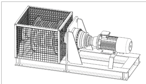
Abbildung 4 Trommelschutzabdeckung PHW
