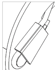
Abbildung 35 Befestigung des Seiles mit Seilkeil
