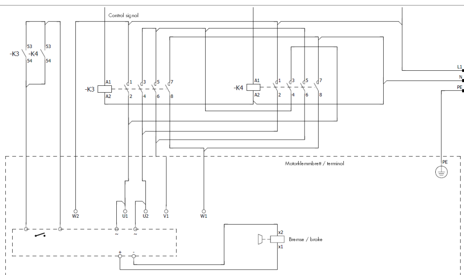
Abbildung 29 Anschluss-Beispiel 230V-Motor
