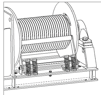
Abbildung 8 Seilandruckrolle PHW
