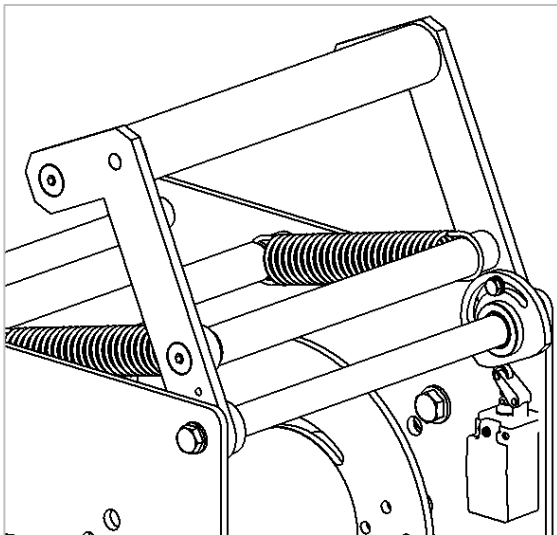
Abbildung 15 Schlaffseilschalter PFW
