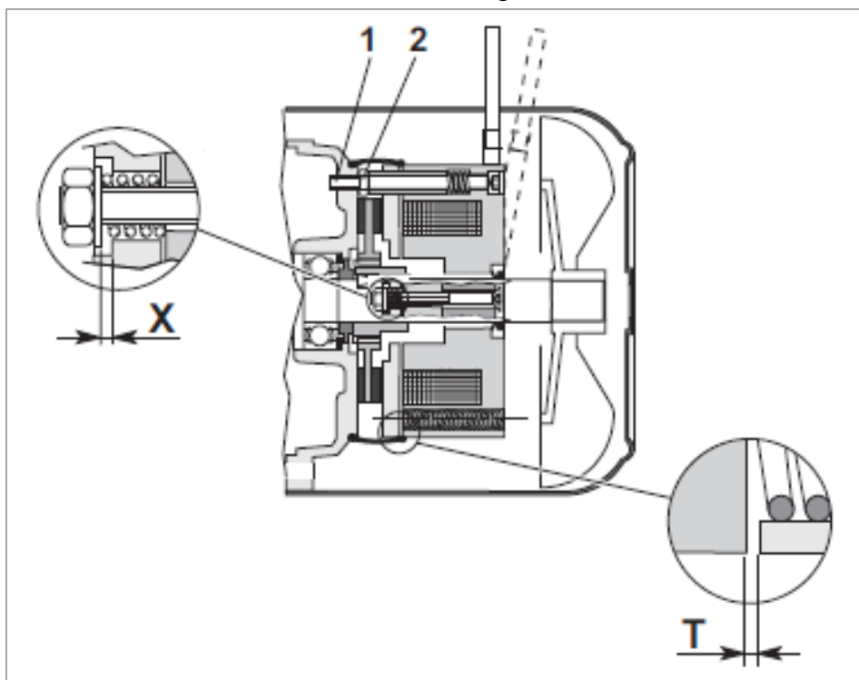
Abbildung 44 Bremsspieleinstellung Typ FD
