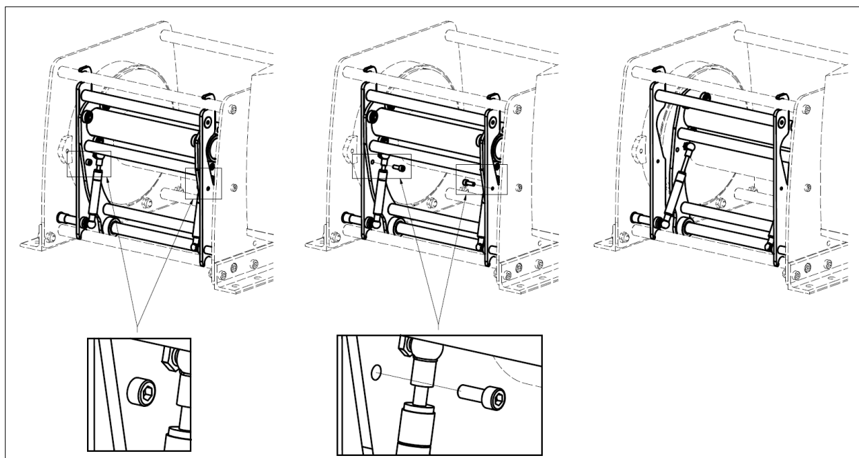
Abbildung 7 Seilandruckrolle
