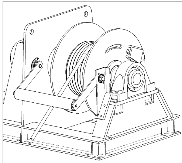
Abbildung 16 Schlaffseilschalter PHW
