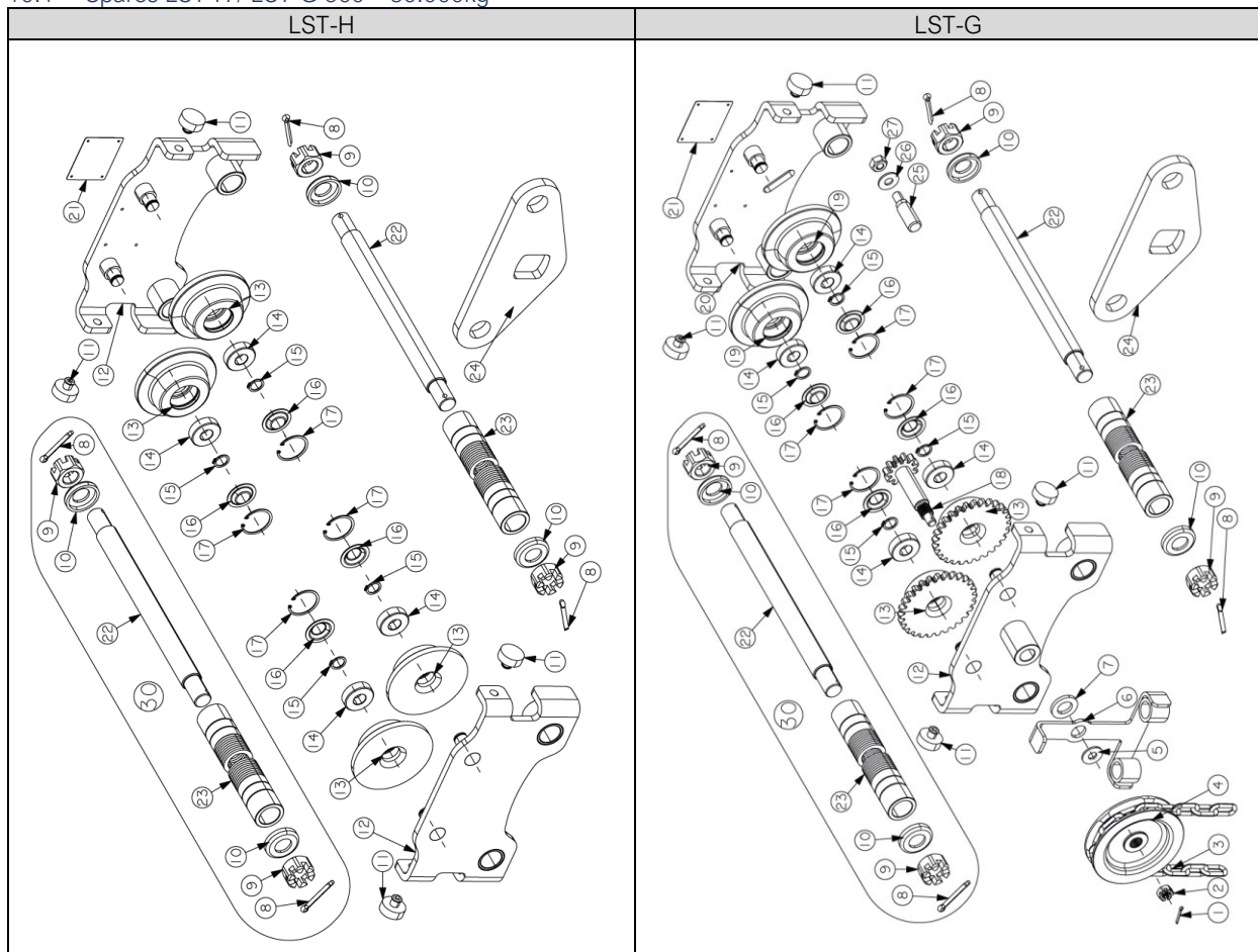
Tafel 6 Spares LST-H / LST-G 500kg – 30.000kg
