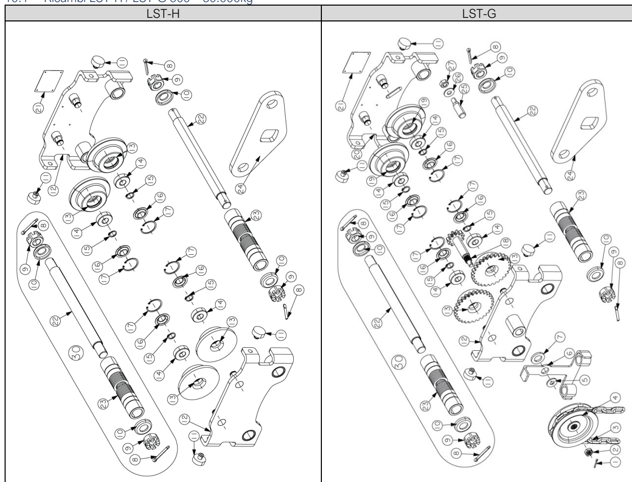
Tavolo 6 Ricambi LST-H / LST-G 500kg – 30.000kg
